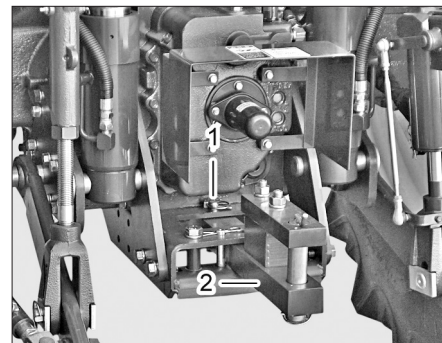
(1) 두부핀 (2) 드로우바
