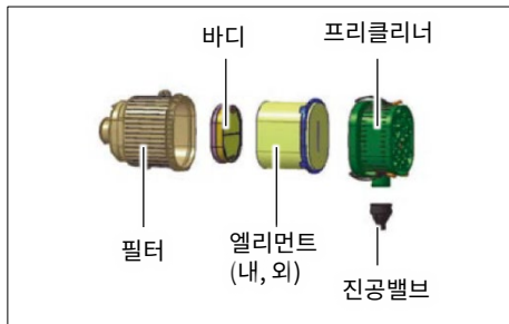
에어클리너
