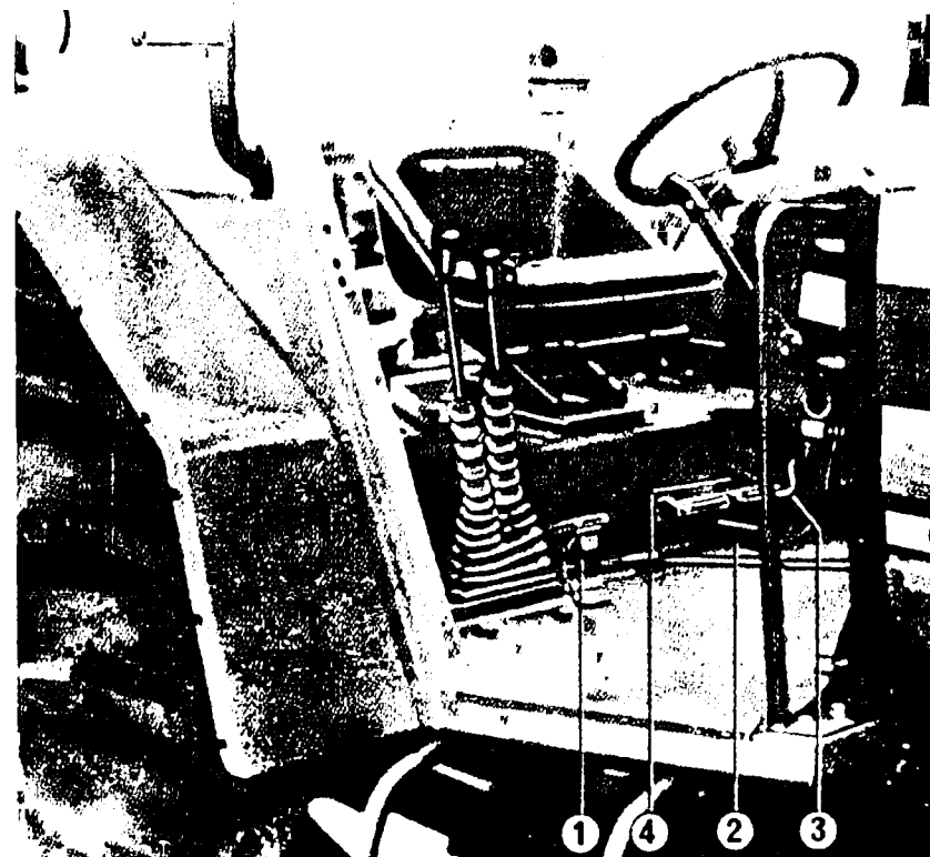
그림 16 운전석 우측
