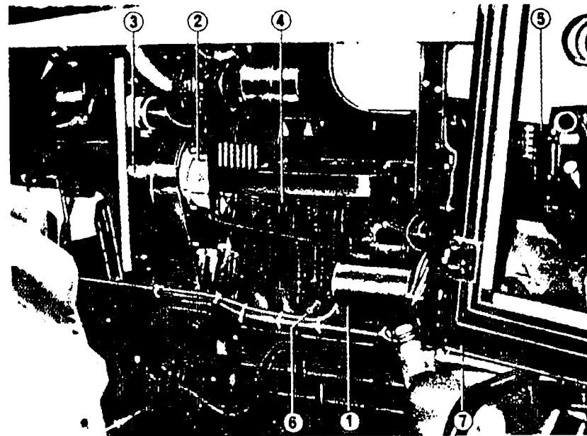
그림 37 엔진 좌측
