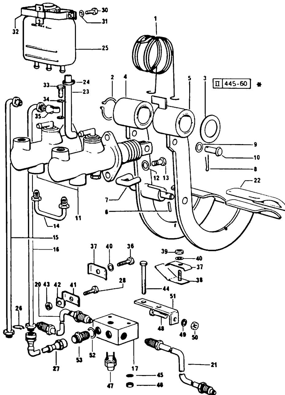
FIG. 64 브레이크 조절관계
