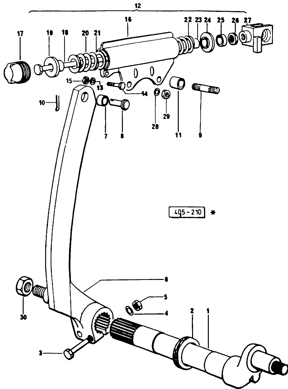
FIG. 210 부하제어센서 관계
