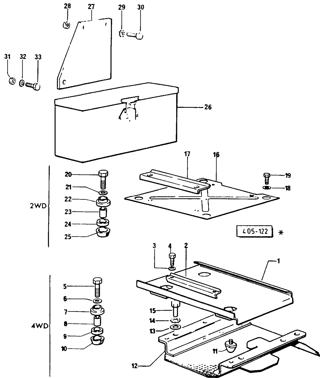
FIG. 122 배터리커버, 공구박스 관계
