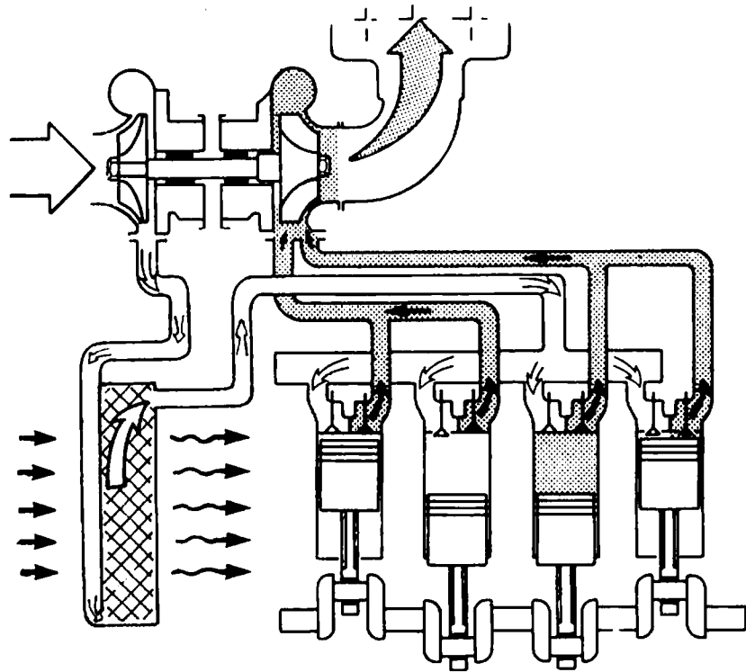
그림 10 터보 차지 개념도
