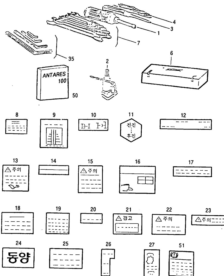
FIG. 232 공구 및 명판관계
