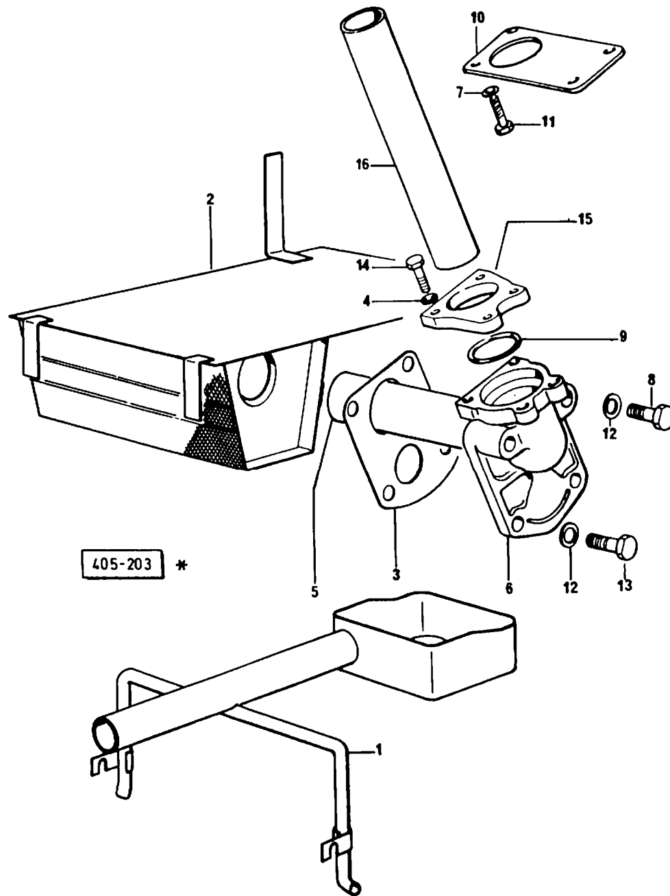
FIG. 203 오일석선 관계
