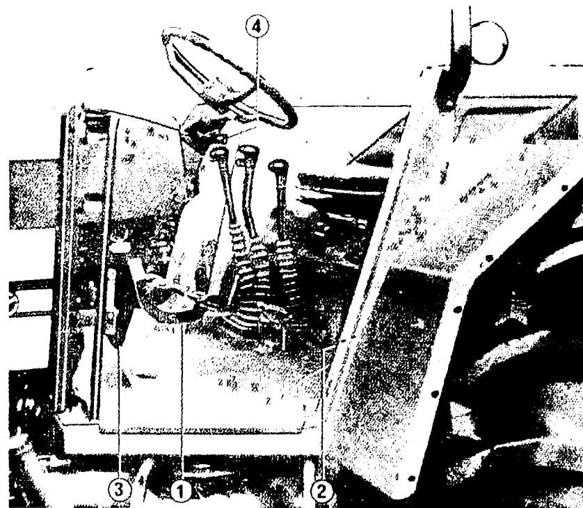
그림 12 운전석 좌측
