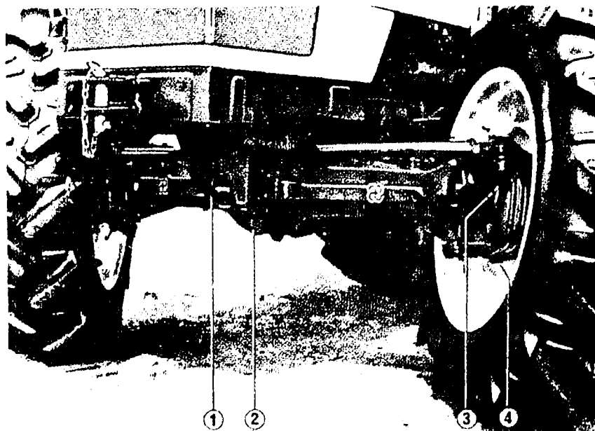
그림 42 앞차축
