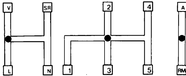
그림 13 기어 변속도
