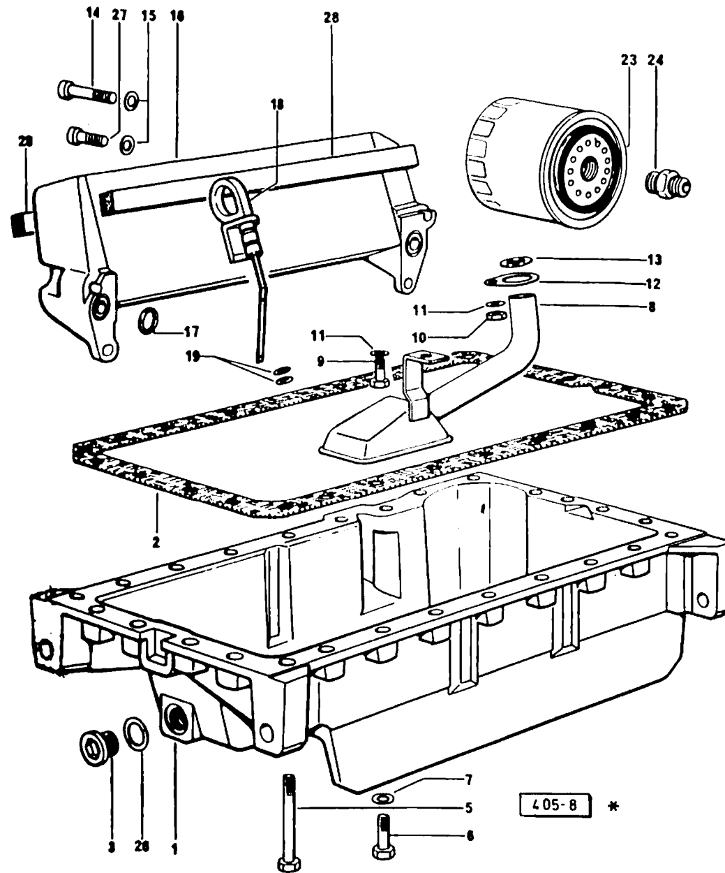
FIG. 8 윤활 관계
