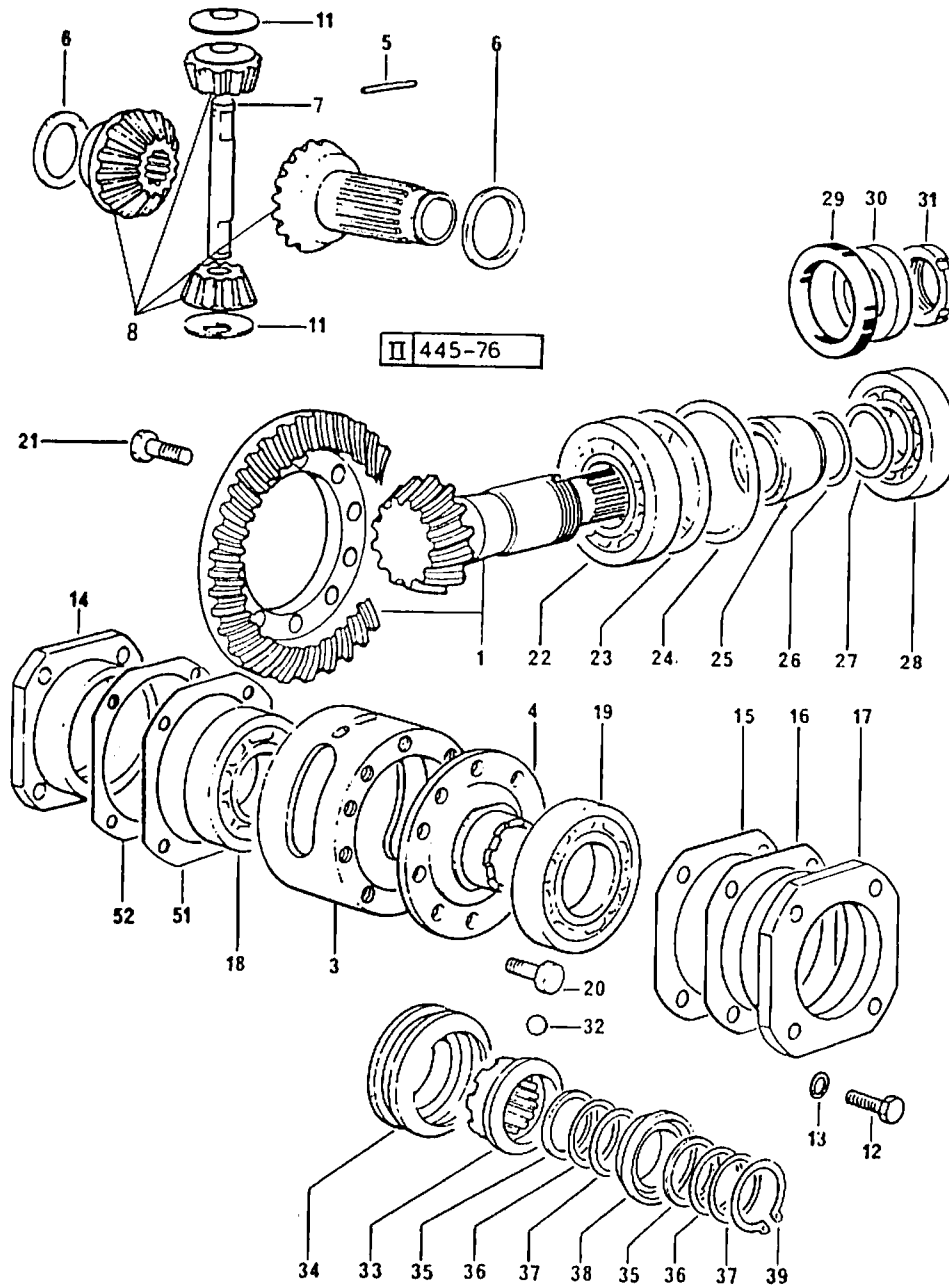
FIG. 79 프론트차동장치 관계
