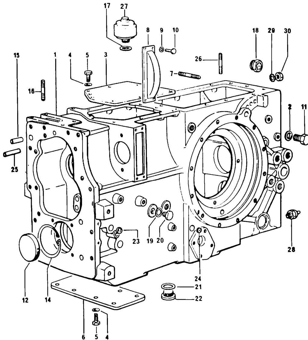
FIG. 34 기어박스 관계
