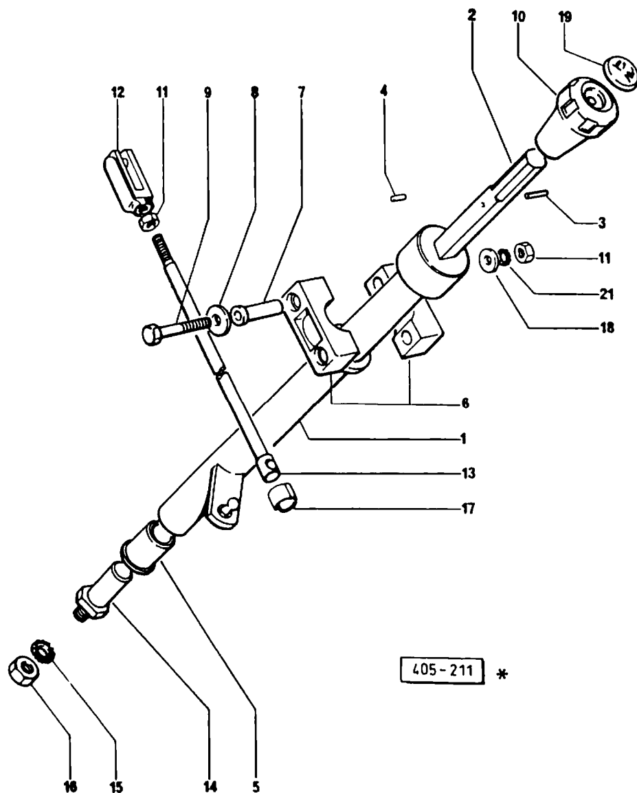
FIG. 211 그라운드 조절관계
