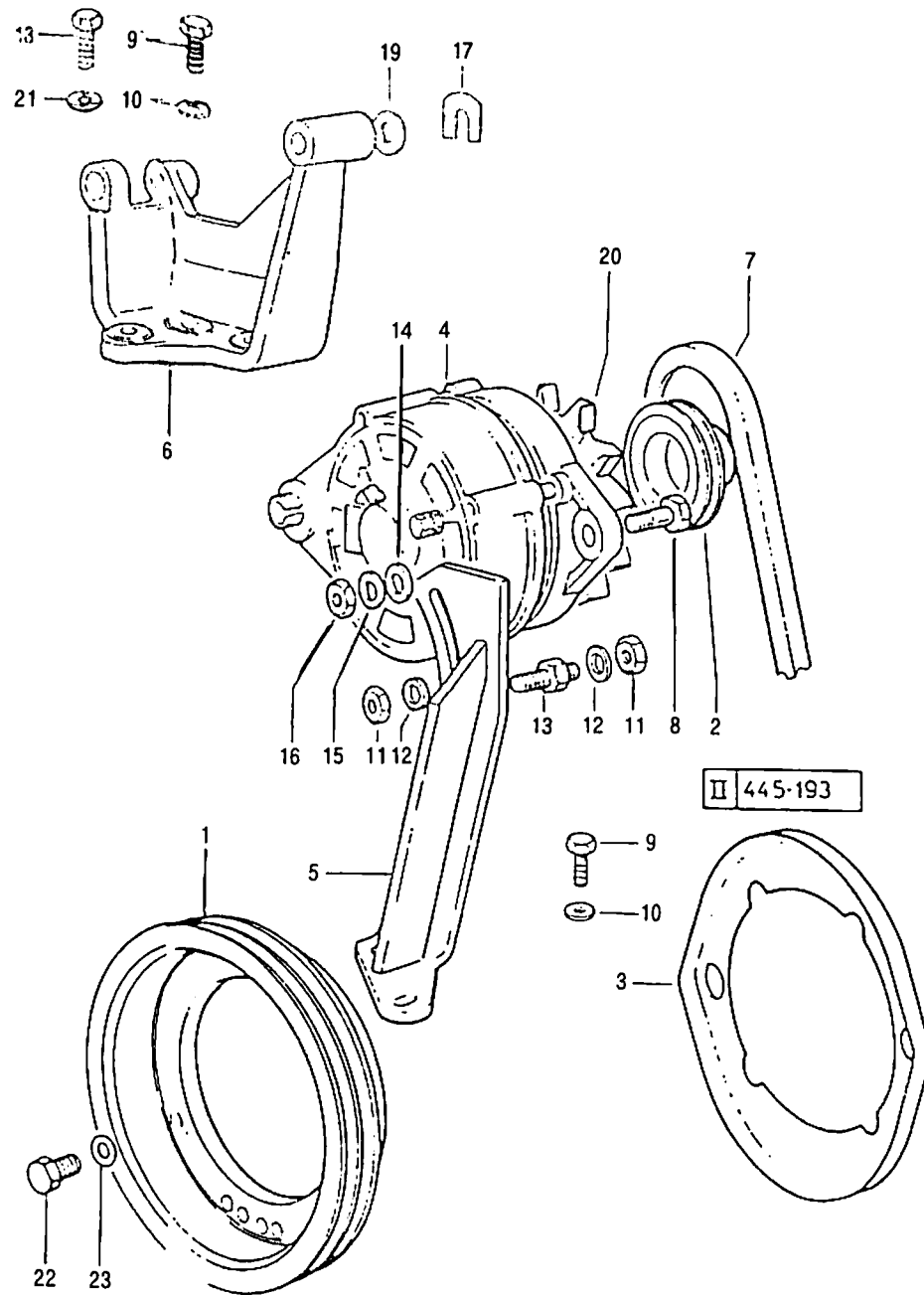
FIG. 196 히터(발전기) 관계
