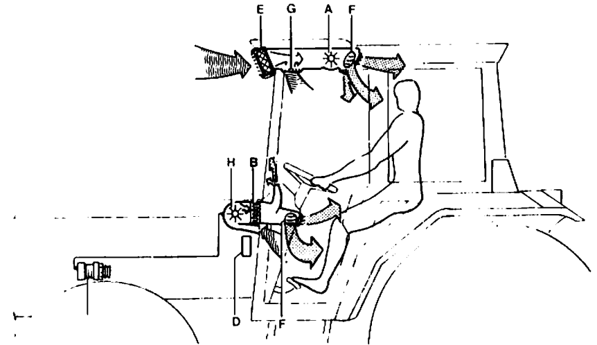
그림 28 난방장치와 송풍장치
