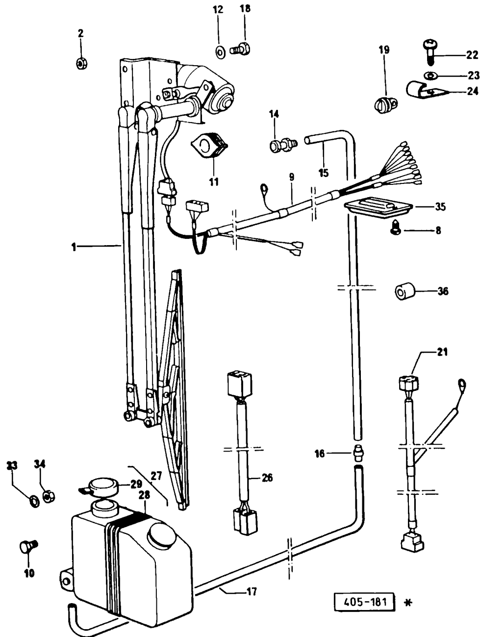
FIG. 181 와이퍼 관계
