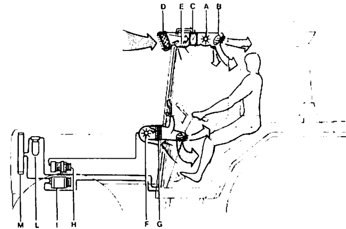
그림 30 냉난방 장치
