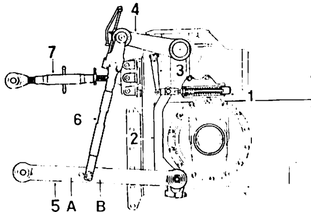
그림 20 트랙터의 승강장치(3점 히치)
