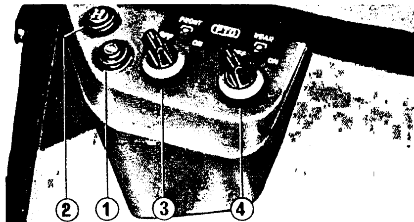
그림 18 P.T.O., 4륜구동 및 차동고정 장치(디프 록) 조정 버튼
