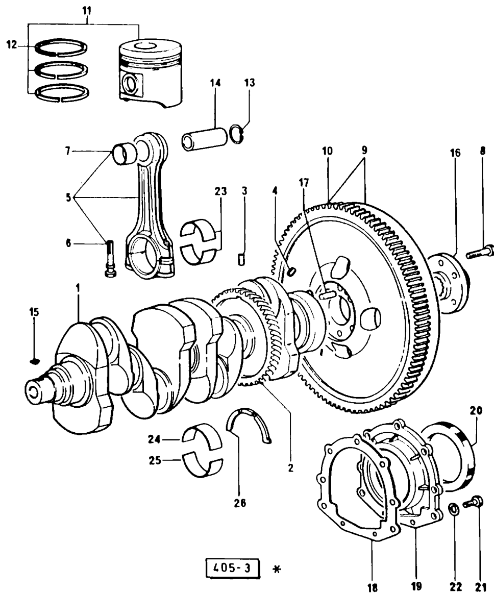
FIG. 3 크랭크축 관계
