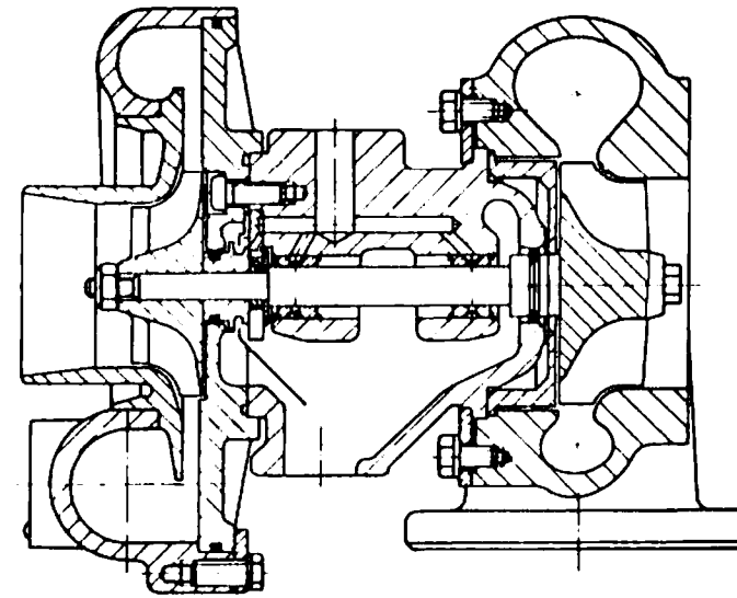
그림 11 터보차저
