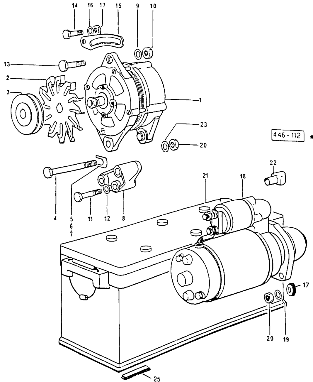
FIG. 160 전기장치 관계
