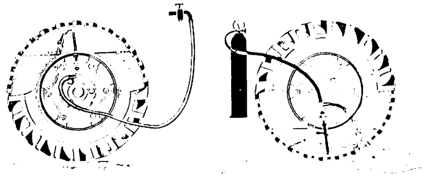
그림 50 타이어의 물 주입 및 배수 방법
