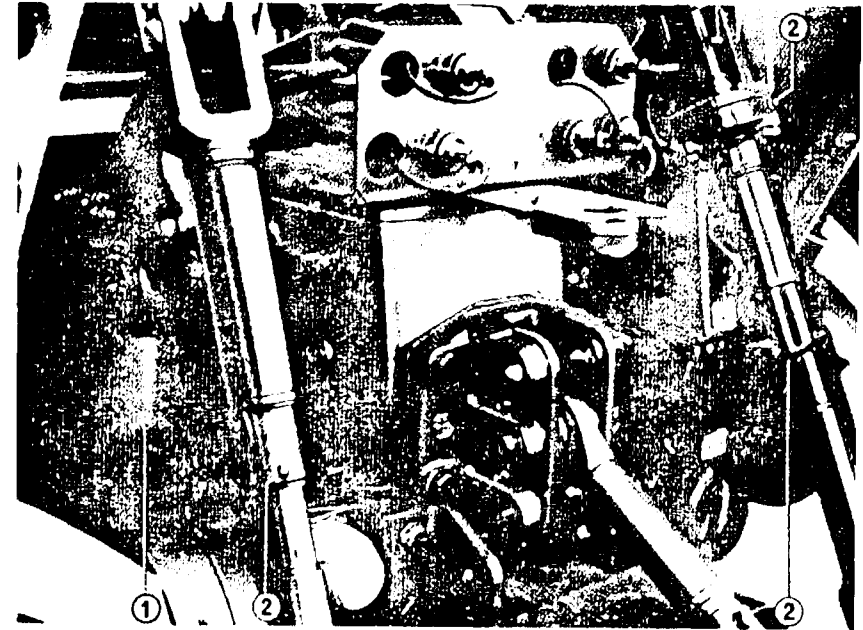
그림 48 부하감지 유압 승강장치
