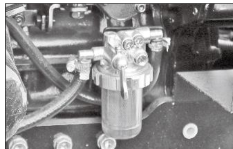
필터(연료) 조합
