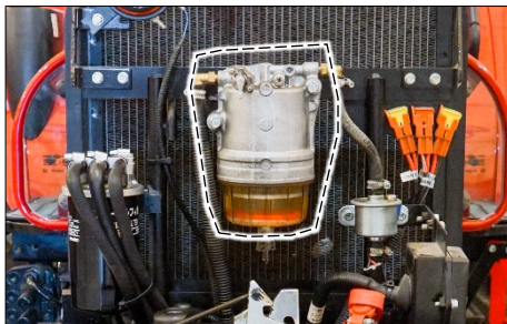
프리 연료 필터
