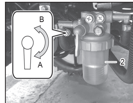
(1) 연료 필터
