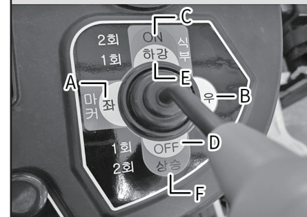
(1) 크로스 레버 (A) 마커(좌) (B) 마커(우) (C) 식부 ON (D) 식부 OFF (E) 식부 하강 (F) 식부 상승
