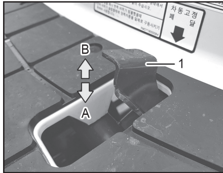
(1) 차동 고정 페달 (A) 차동 고정 (B) 차동 해제
