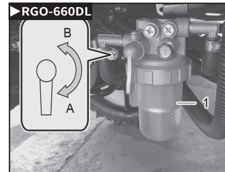
(1) 유수 분리기 (A) 개 (B) 폐
