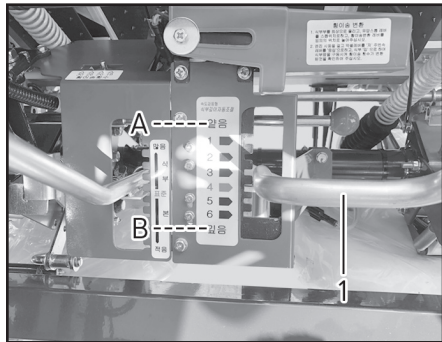
(1) 식부깊이 조절 레버
