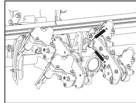
▶각조 클러치 암 회동 지점
