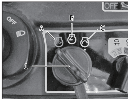
(1) 키 스위치 (A) OFF (B) ON (C) START
