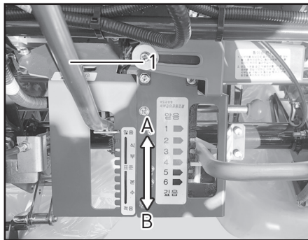
(1) 식부분수 조절 레버
