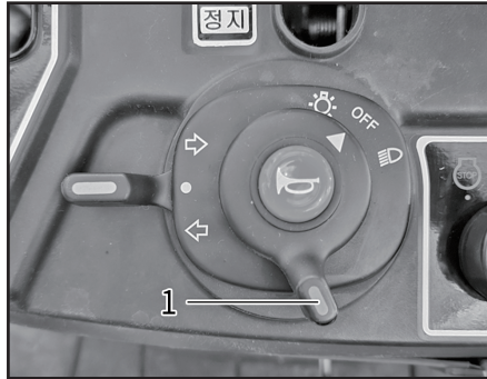
(1) 라이트 스위치
