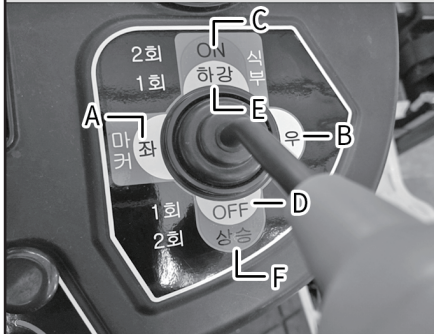
(1) 크로스 레버 (A) 마커(좌) (C) 식부 ON (E) 식부 하강 (B) 마커(우) (D) 식부 OFF (F) 식부 상승
