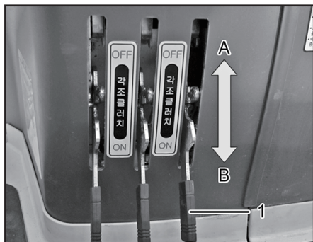
(1) 각조 클러치 레버 (A) 「OFF」 식부조 정지 (B) 「ON」 식부조 작동
