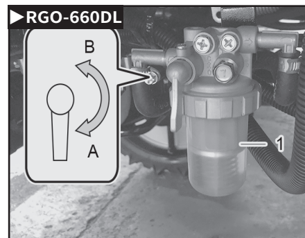
(1) 유수 분리기
