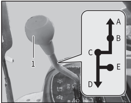
(1) 주변속 레버
