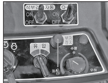
(1) 부저정지 스위치
