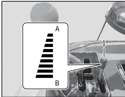
(1) 액셀 레버
