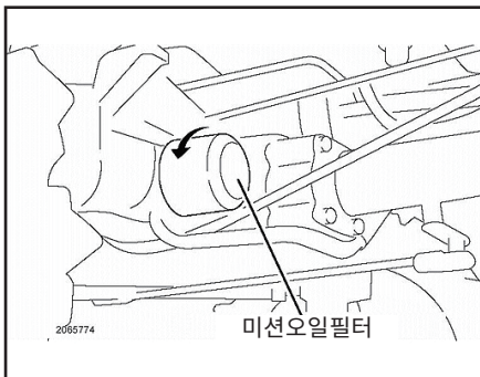
(1) 미션오일 필터
