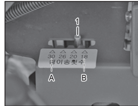
(1) 횡 이송 변환 레버
