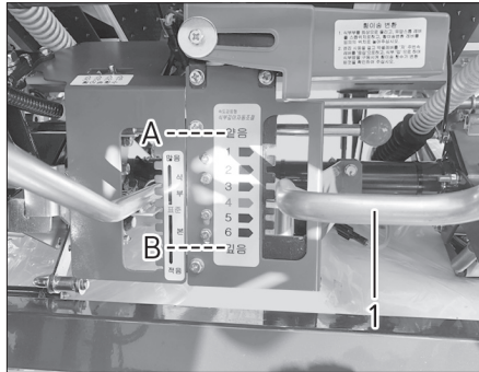
(1) 식부깊이 조절 레버 (A) 얇음 (B) 깊음
