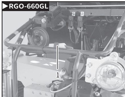
(1) 퓨즈 블링크
