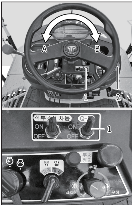
(1) Q-턴 스위치 (2) 크로스 레버 (A) 좌회전 (B) 우회전
