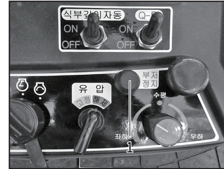
(1) 부저 정지 스위치
