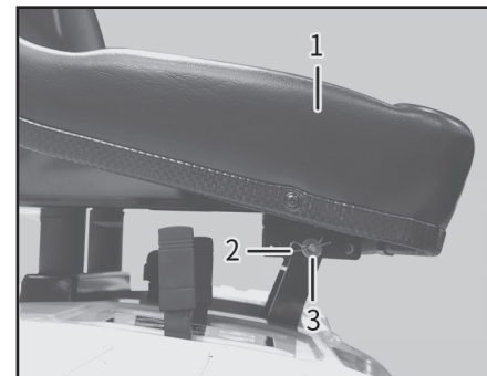
(1) 의자
