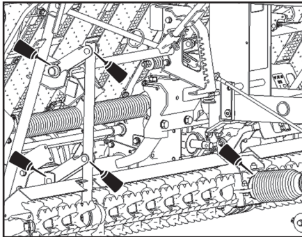
▶써레 프레임 링크 / 써레 높이 조절 레버 지점부
