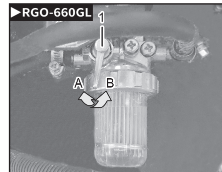
(1) 연료코크 레버
