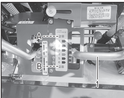
(1) 식부깊이 조절레버
