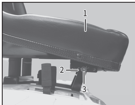
(1) 의자 (2) 스넵핀 (3) 지점핀
