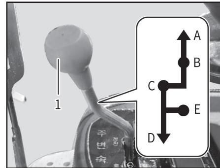
(1) 주변속 레버
