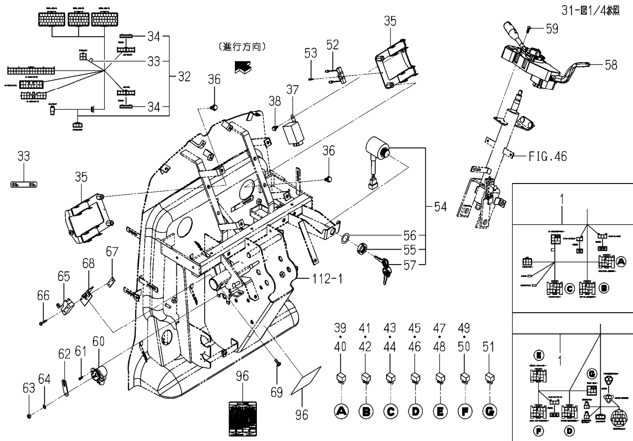
1842-096-100-0A FIG.084 ELC. 시스템 (메인) 關係 (TJW1233-D型) (圖2/4)
