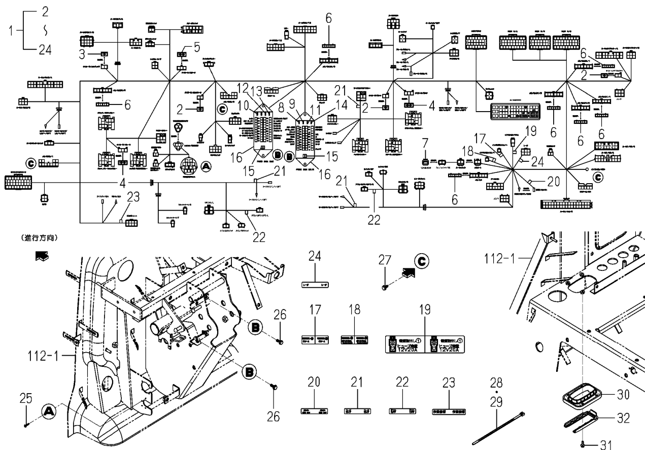
1842-096-100-0A FIG.086 ELC. 시스템 (메인) 關係 (TJW1153-X型) (圖1/4)
