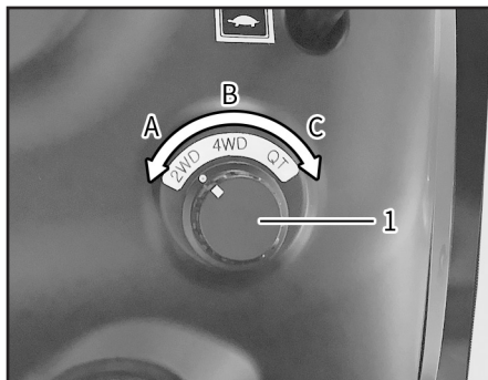
(1) 주행구동 스위치
