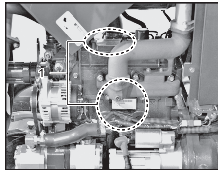
(1) 엔진번호
