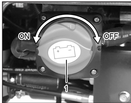
(1) 전원차단 스위치
