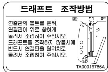
(21) 부품번호: TA00016786
