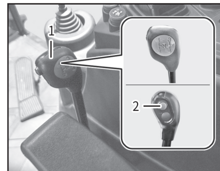
(1) 주변속 레버 (2) De-clutch 버튼 (디클러치)
