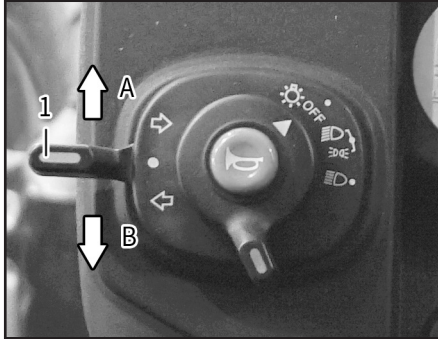
(1) 방향지시등 스위치 (A) 우측 방향지시등 (B) 좌측 방향지시등
