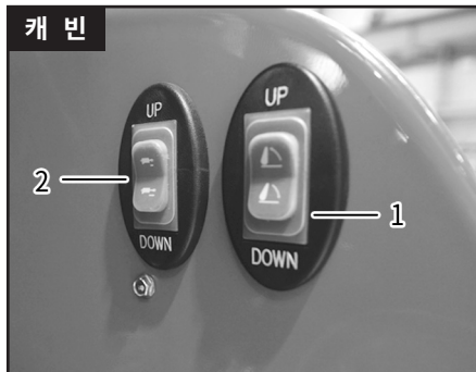
(1) 유압 승강 실린더 (2) 수평제어 실린더
