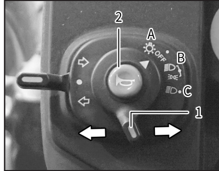
(1) 전조등 스위치 (2) 혼 스위치 (A) OFF (B) 하향등 (C) 상향등
