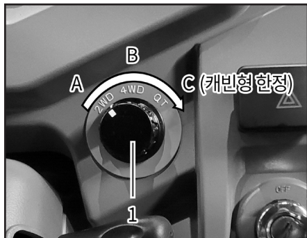
(1) 전륜구동 스위치 (A) 2WD (B) 4WD (C) QT (캐빈형)
