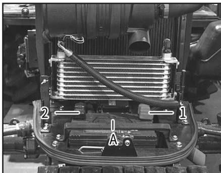
(1) 붉은 붉은선(+) (2) 접지선(-) (A) 점검창 (B) 나비볼트
