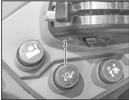
(1) 회전상승 스위치
