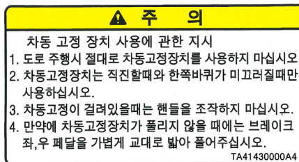
(20) 부품번호: TA41430000
