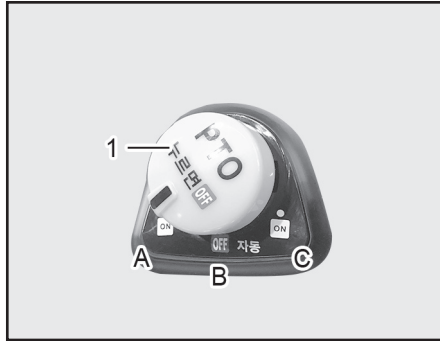
(1) PTO 절환 스위치 (A) ON(독립) (B) OFF (C) ON(연동)
