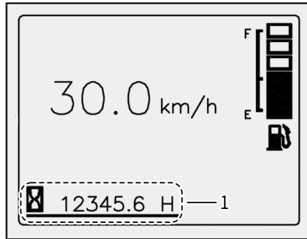
(1) 사용시간 적산계
