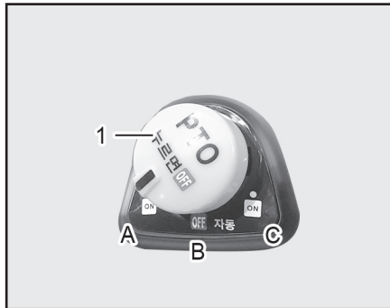
(1) PTO 작동 스위치 (A) ON(독립) (B) OFF (C) ON(연동)
