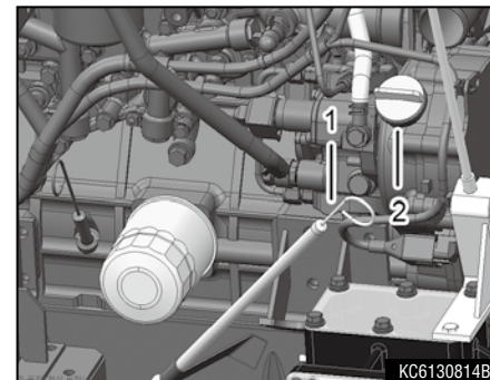
(1) 검유 게이지 (2) 급유구
