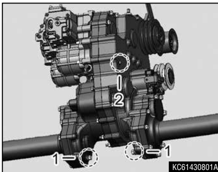
(1) 드레인 플러그 2개소 (2) 검유 플러그(항색표시)
