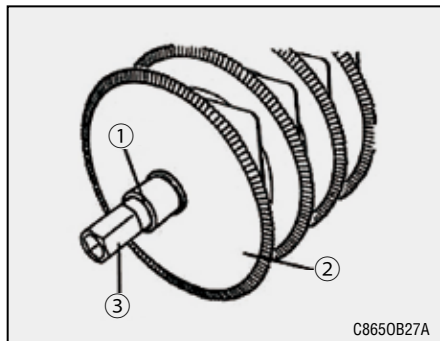
(1) R형 스냅링 S30 (2) 회전날 (3) 파이프 축
