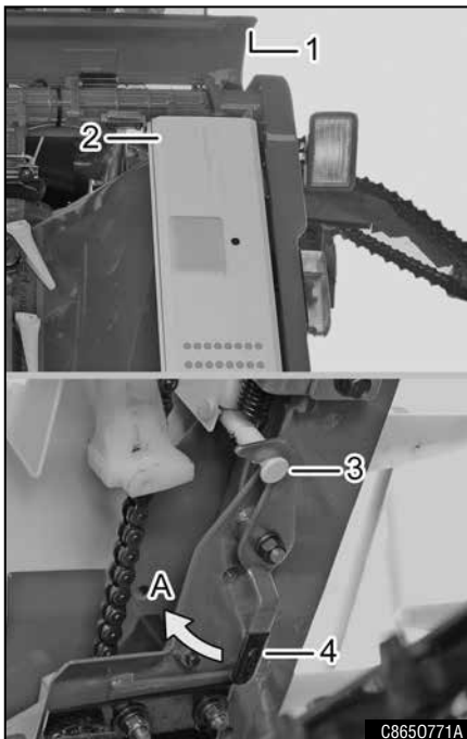
(1) 프론트 게이트 (2) 인기케이스 커버 (3) 케이스 고정핀 (4) 케이스 고정캡 핸들 (A) 언다
