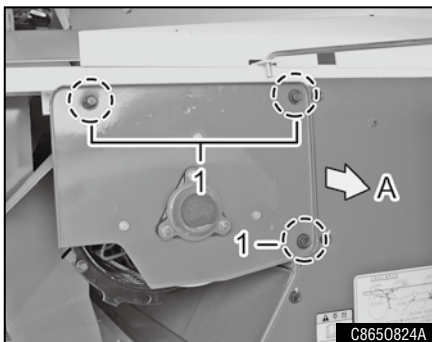
(1) M10 볼트
