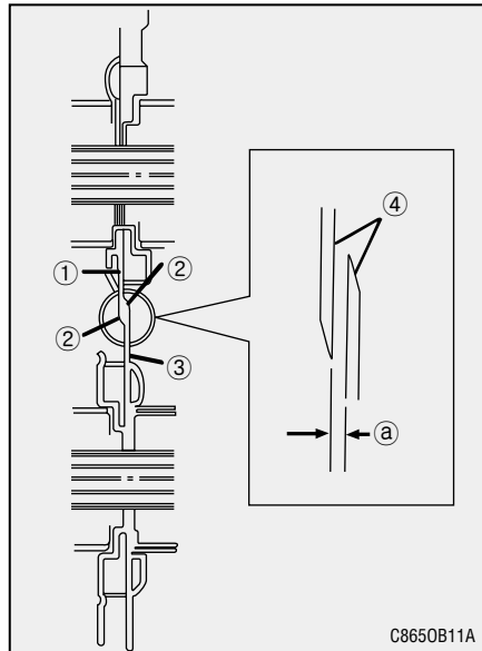
(1) 저속날
