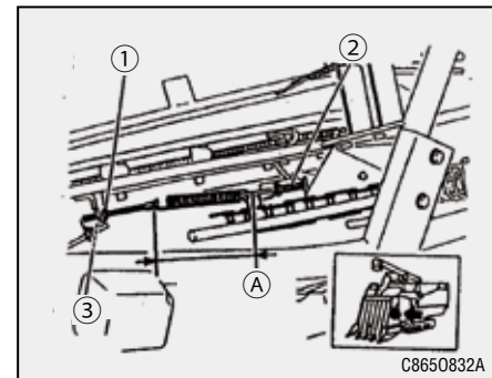
(1) 고정너트 (2) 스톱퍼 볼트 (3) 조절너트 (A) 스프링 후크 길이: 185~189mm(스트링 틈새1.2~1.4mm) 텐션 스프링 후크 길이를 185~189mm(스트링 틈새1.2~1.4mm)로 조절하십시오.
