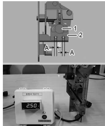
(1) 예취 승강 위치센서 (2) 위치 센서 브라켓
