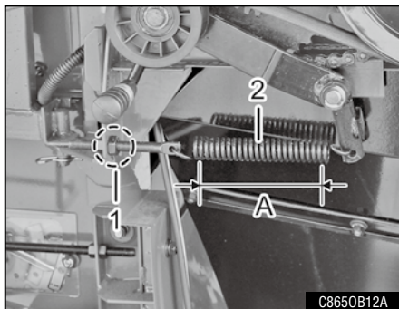
(1) 텐션볼트 (2) 텐션 스프링 (A) 140 \pm 2\text{mm}
