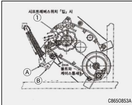
(1) 피드체인 케이스
