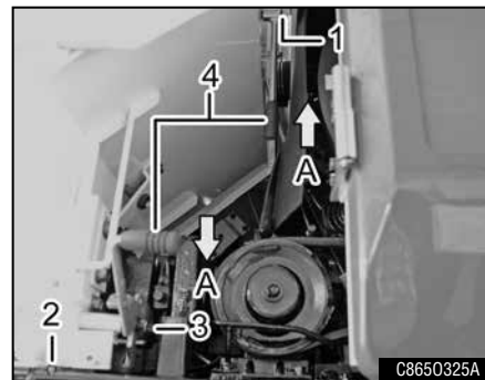
(1) 로크축 (2) 고정볼트 (3) 고정축 (4) 고정레버 (A) 누름
