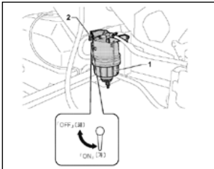
(1) 유수분리기 (2) 코크
