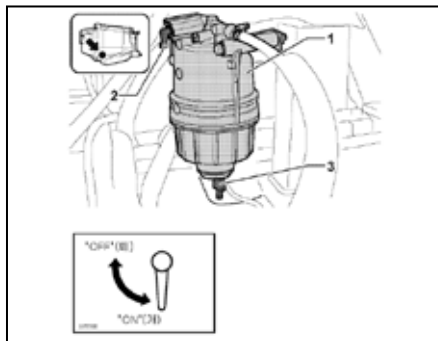
(1) 유수분리기 (2) 코크 (3) 드레인플러그
