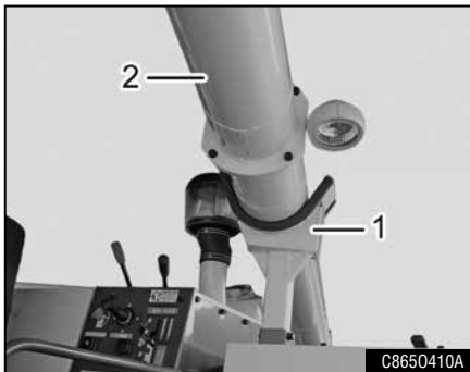
(1) 오거 받침대
