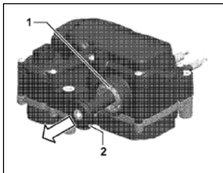
(1) 필터엘리먼트 (2) 이퀄라이징엘리먼트
