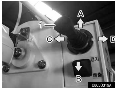
(1) 배출오거 크로스 레버
