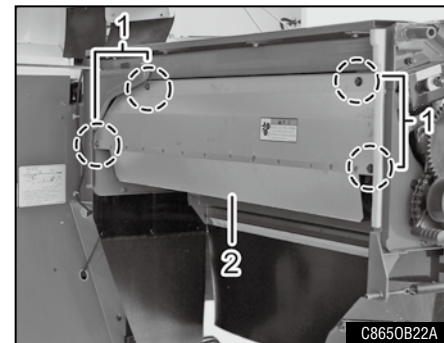
(1) 볼트 (2) 절단 가이드판
