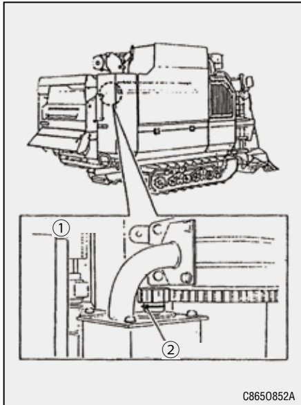
(1) 오거회동 모터
