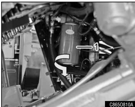
(1) HST 필터 (A) 좌로 돌려서 빼낸다.
