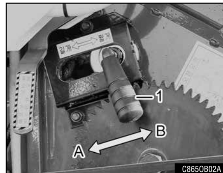
(1) 절단치수 절환레버
