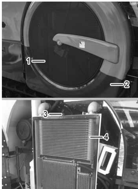
(1) 오토 스크린 (2) 엔진룸 (3) 손잡이 볼트 (4) 라디에이터 스크린
