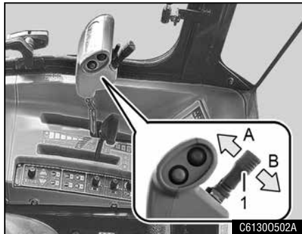
(1) 공급깊이 스위치
