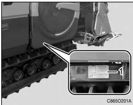
(1) 형식명과 제조번호
