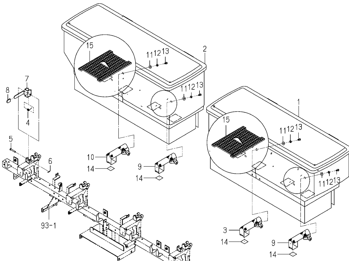
Fig.095 Hopper(Fertilizer)system
