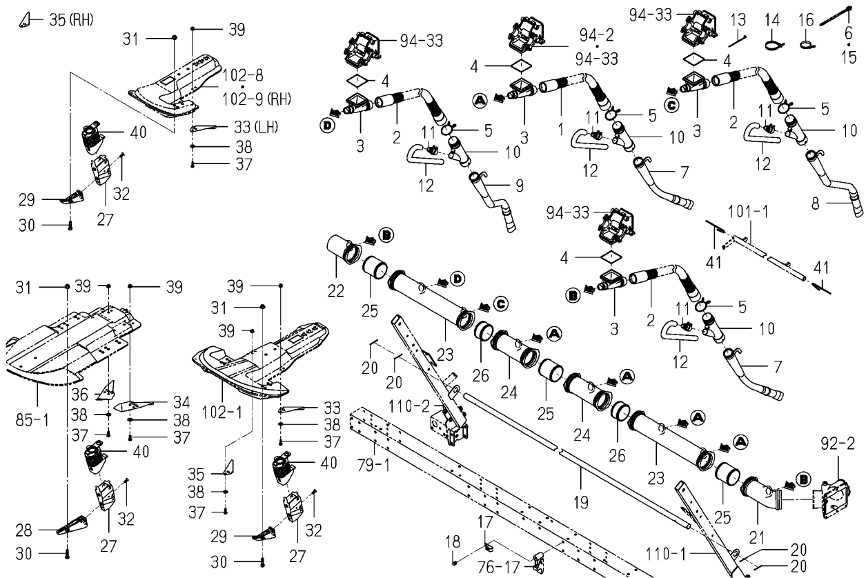
Fig.096 Piping(Fertilizer)system
