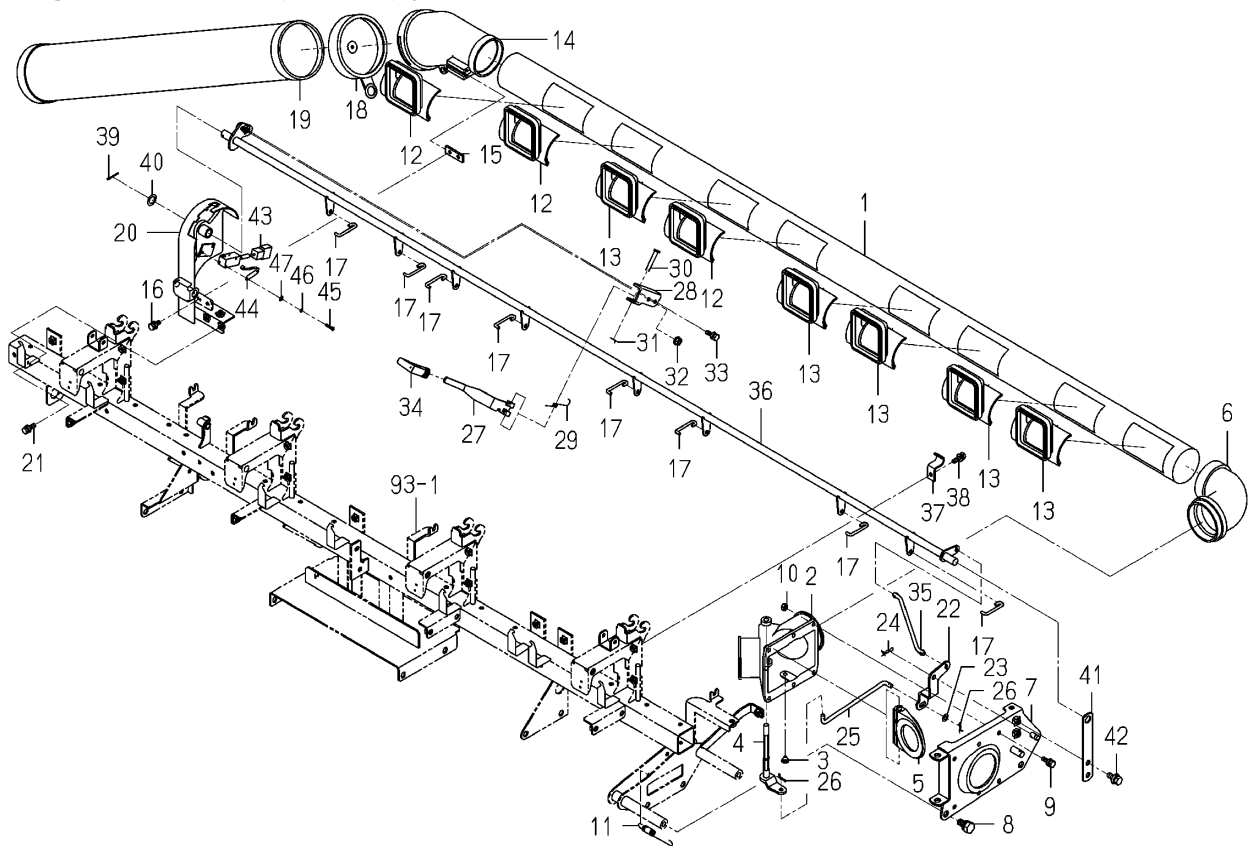
Fig.092 Air Chamber(Fertilizer)system
