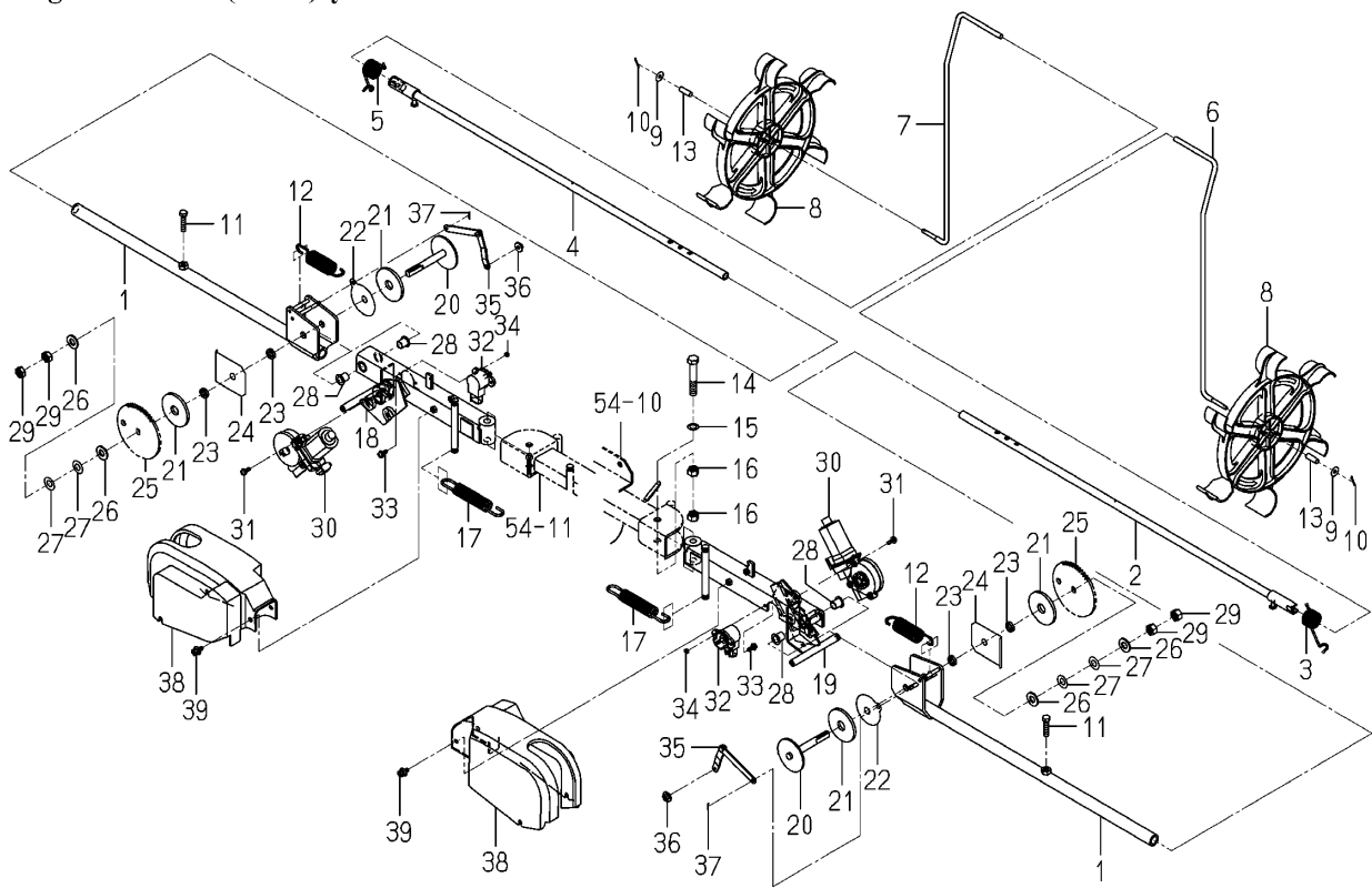
Fig.062 Marker(Front)system
