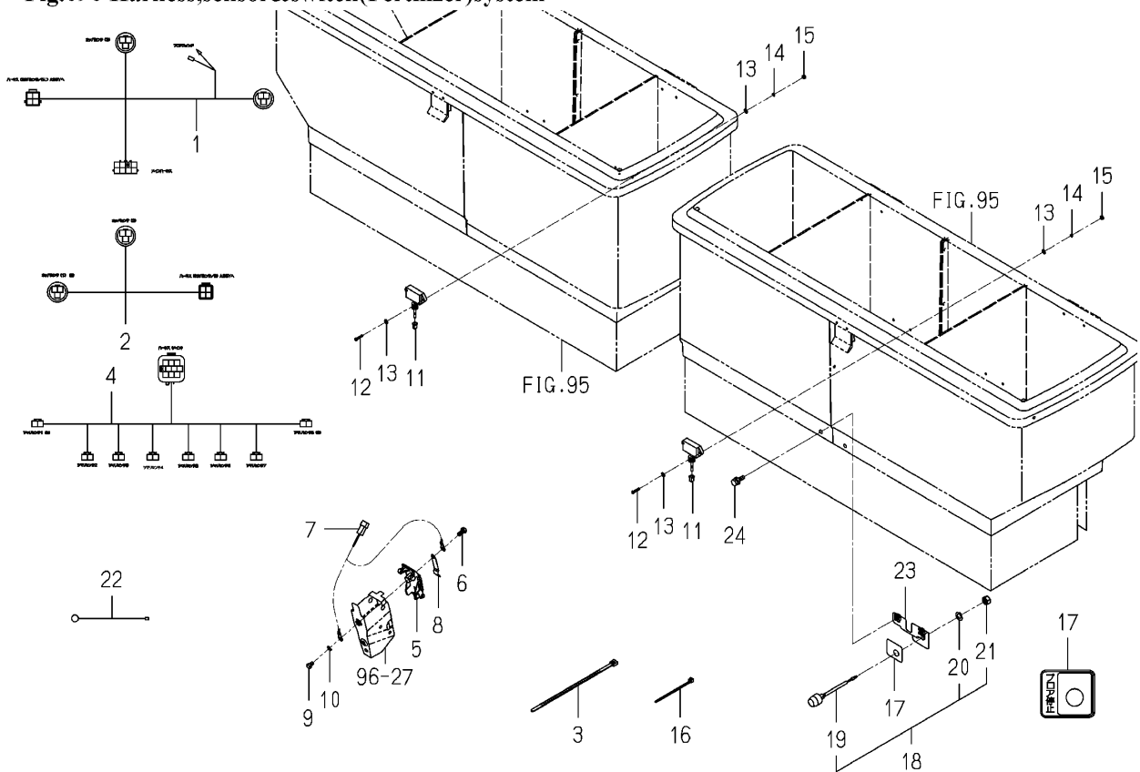
Fig.090 Harness,sensor&amp;switch(Fertilizer)system
