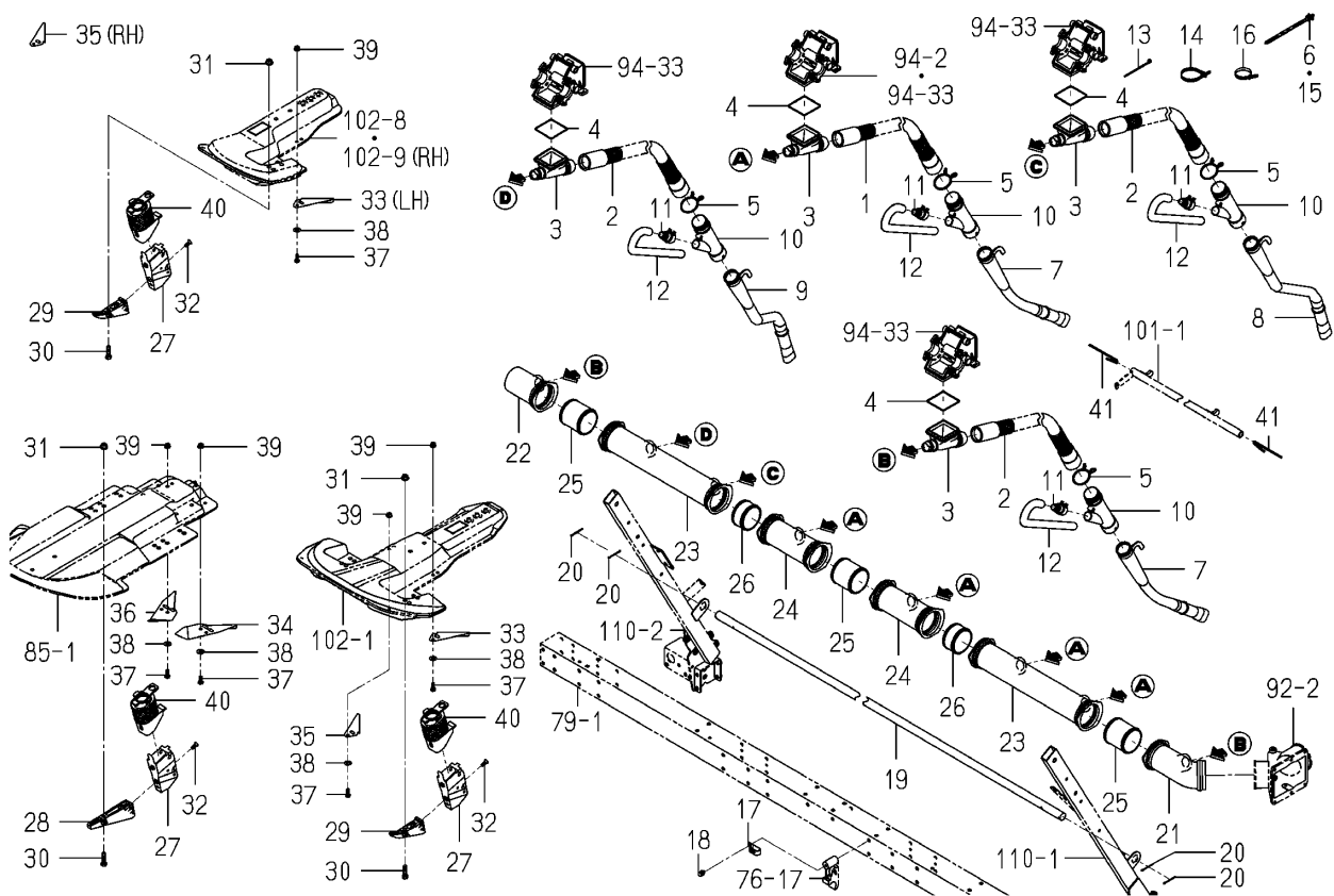
Fig.096 Piping(Fertilizer)system
