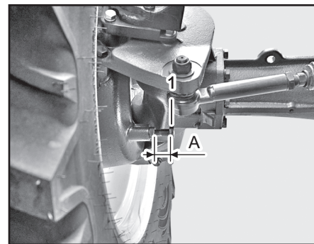
(1) 전차축 스톱퍼 볼트
