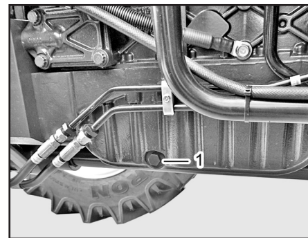
(1) 퇴유 플러그
