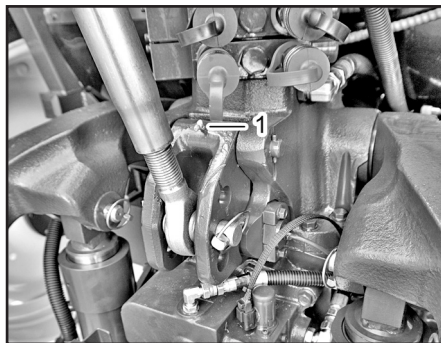
(1) 토크 링크
