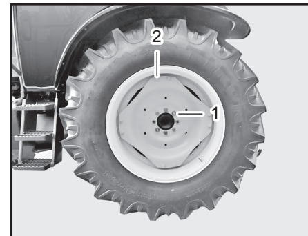
(1) 휠 너트 (2) 림 볼트
