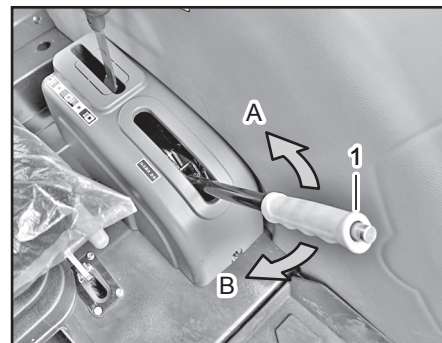
(1) 주차브레이크 레버 (A) 잠금 (B) 해제
