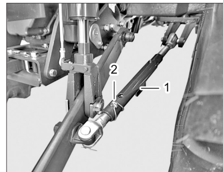
(1) 스테빌라이저바 (2) 링핀 조합
