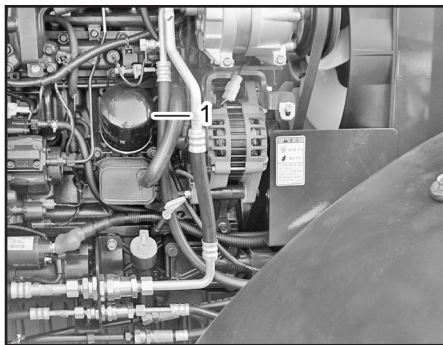
(1) 오일필터 카트리지
