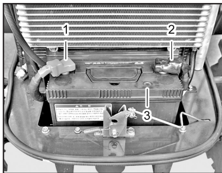
(1) 붉은 붉은선(+) (2) 접지선(-) (3) 점검창
