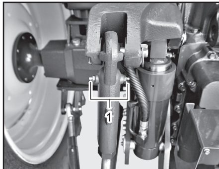
(1) 리프트 링크(좌)
