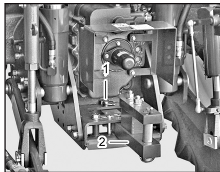
(1) 두부핀 (2) 드로우바
