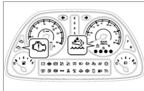
<요소수 공급 장치(S.M.)이외의 다른 문제점 (SCR) 발생시>
