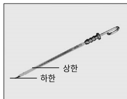
<레벨 게이지>
