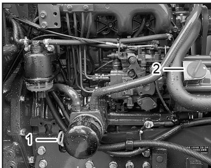
(1) 오일 게이지
