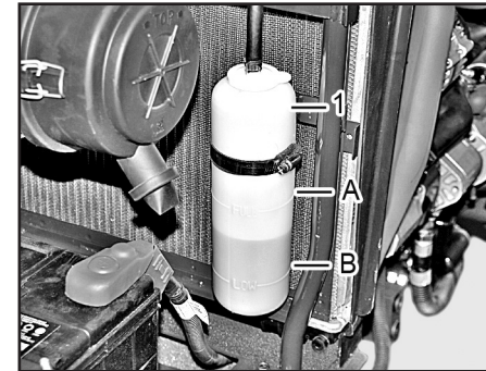
(1) 냉각수 보조탱크
