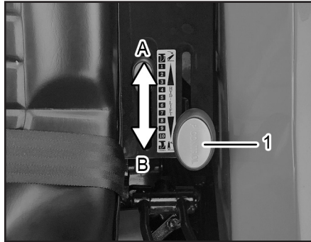
(1) 위치제어 레버 (A) 하강 (B) 상승
