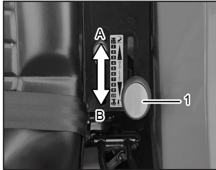
(1) 위치제어 레버
