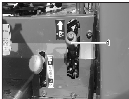
(1) 주차브레이크 레버
