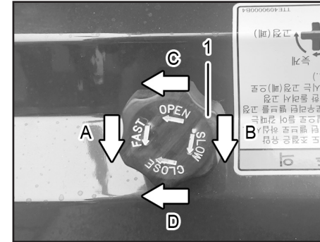
(1) 스톱/슬로우 리턴 밸브
