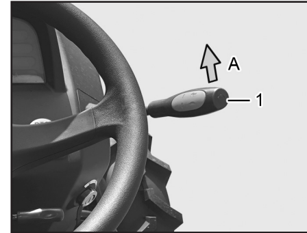
(1) 액셀 레버 (A) 엔진 RPM 증가
