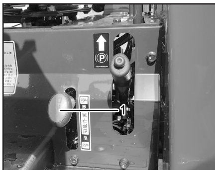
(1) 전륜구동 레버
