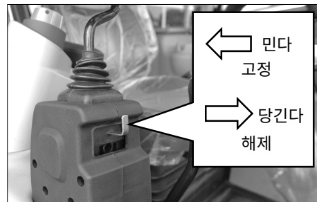
<조이스틱 레버 안전 장치>
