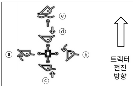
<조이스틱 레버 방향에 따른 동작>
